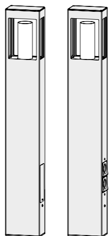
H1100. W170. D100
